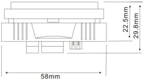
正视图
